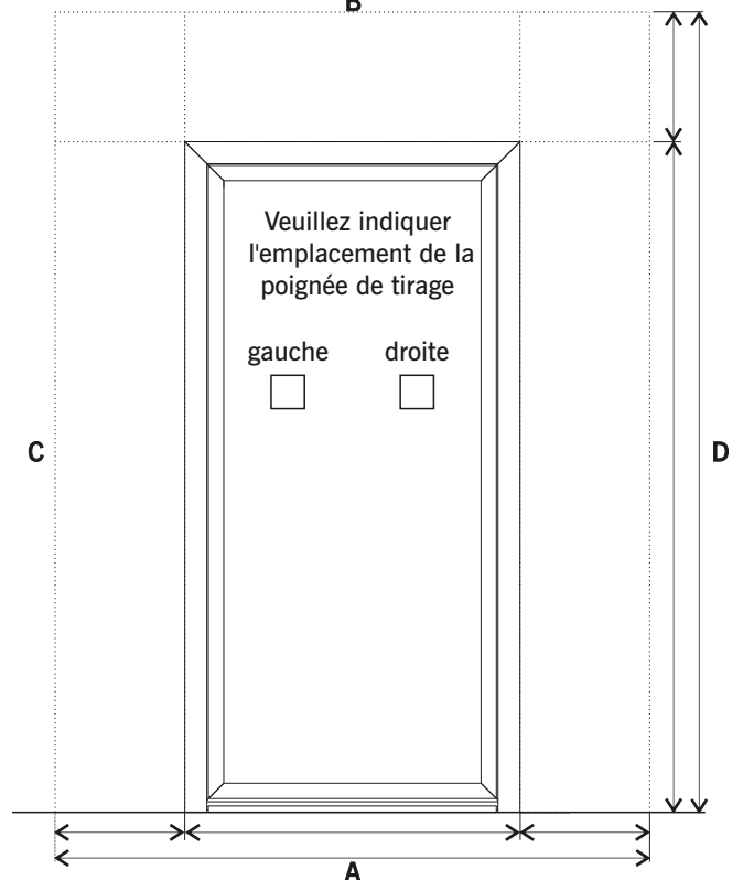
La affichage schématique de porte - Regard extérieur
